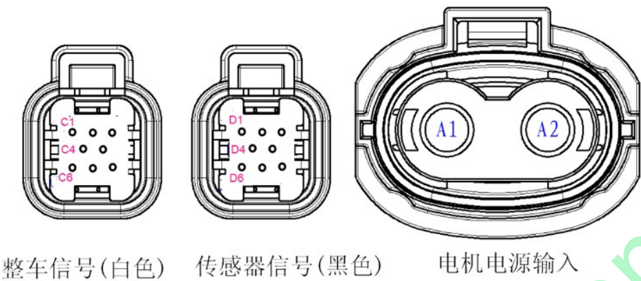
图 2-2 EPS 线束端引脚定义（测试端视图） 表 2-1 EPS 电子控制单元板端引脚定义
